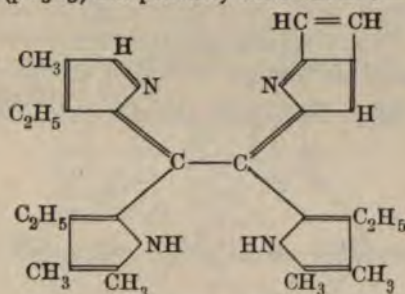
Ætioporphyrin, \text{C}_{31}\text{H}_{36}\text{N}_4 .
